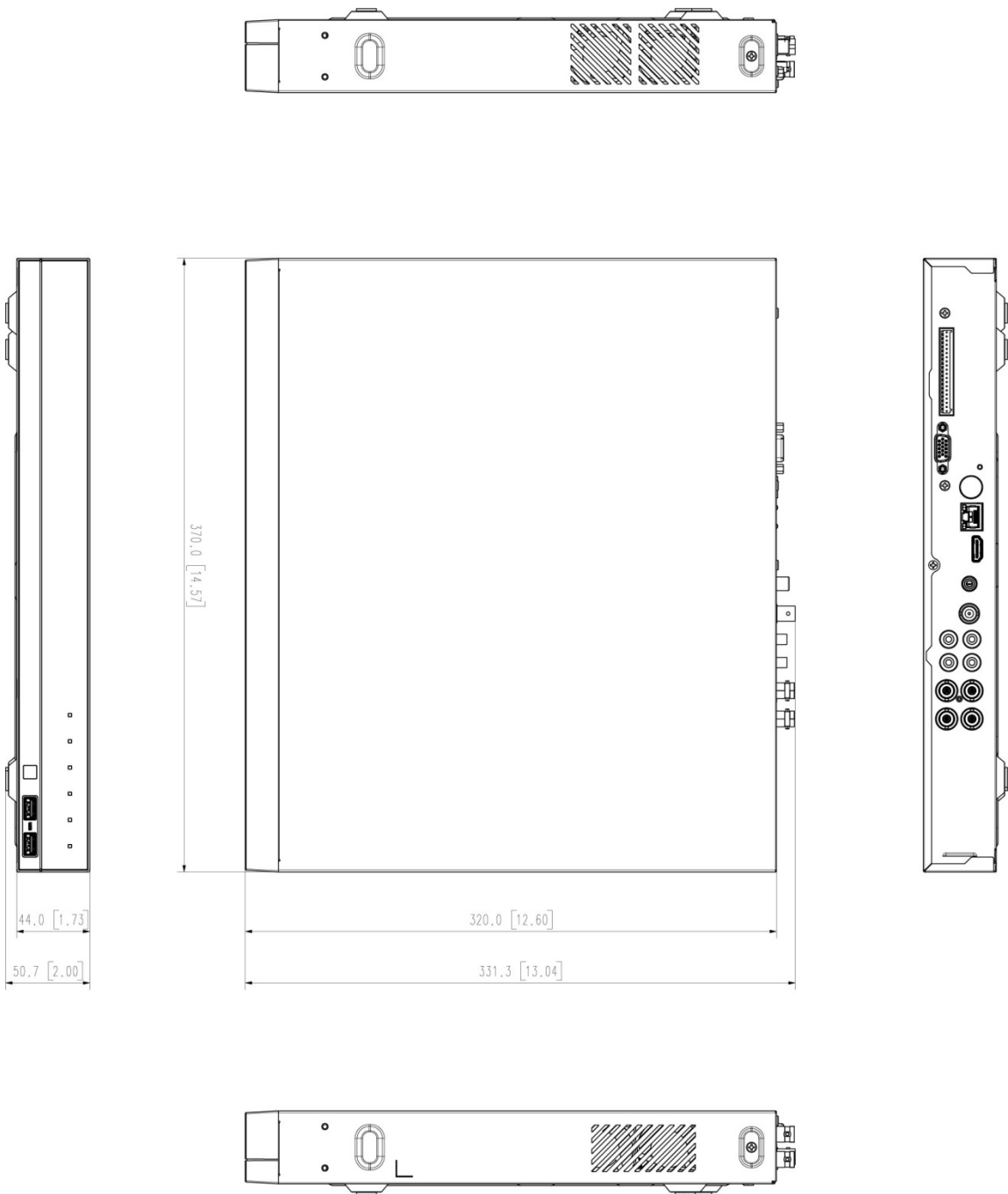
Apariencia del diseño HRX-421 Unidad: mm
